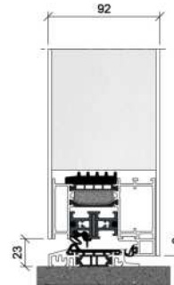
KÖSTER ADVANCE 88 mit einem 75 mm Blendrahmen
